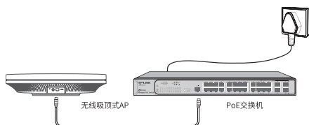
图2-1 PoE供电示意图
